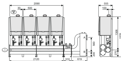
KIT CASCATA MULTI-RE 4 LINEA DN65
