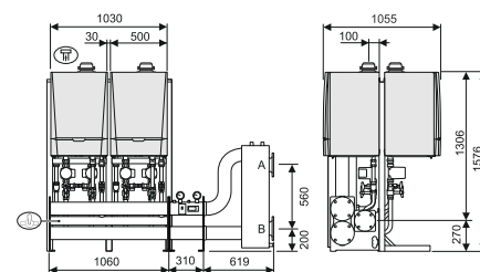
KIT CASCATA MULTI-RE 6 FRONTE/RETRO DN100
