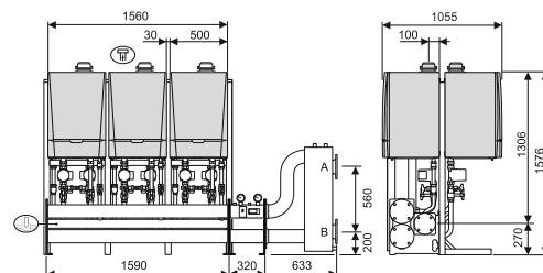
KIT CASCATA MULTI-RE 6 FRONTE/RETRO DN100
