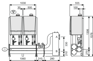
KIT CASCATA MULTI-RE 3 LINEA DN65
