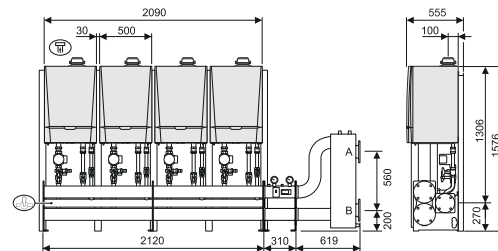
KIT CASCATA MULTI-RE 4 FRONTE/RETRO DN65
